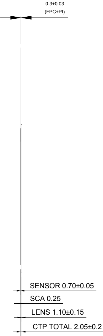
侧视图
