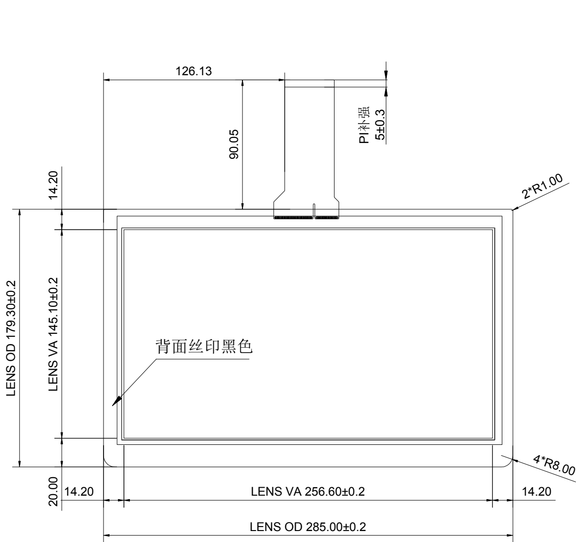
正视图
