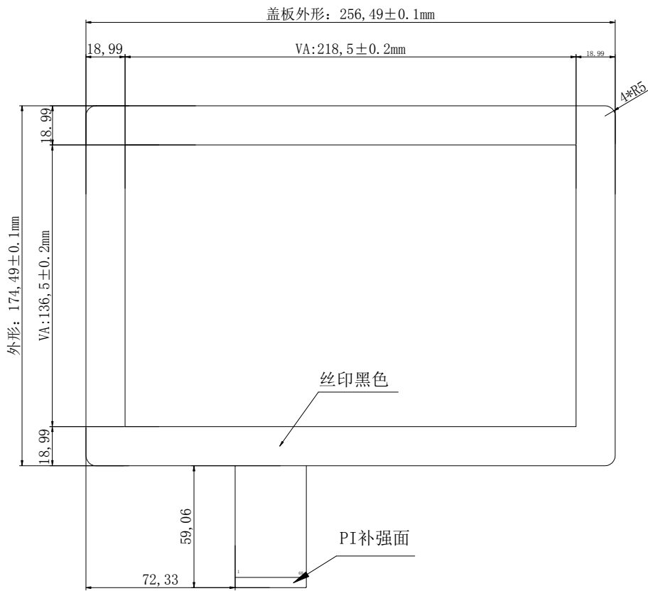
正视图
