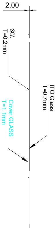
侧视图
