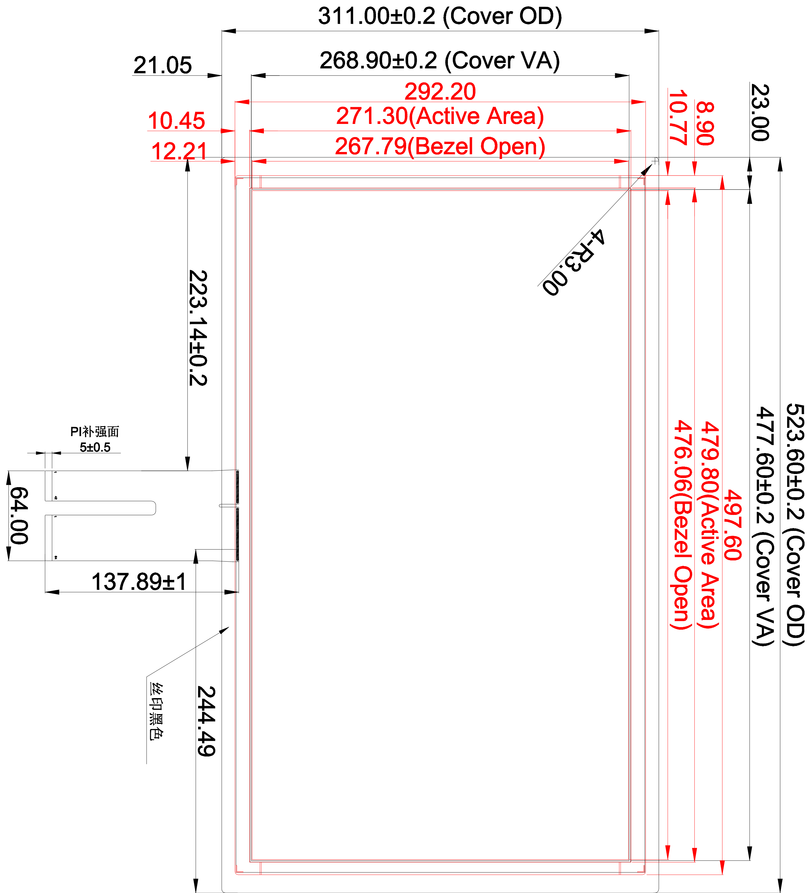
前视图 1:1
