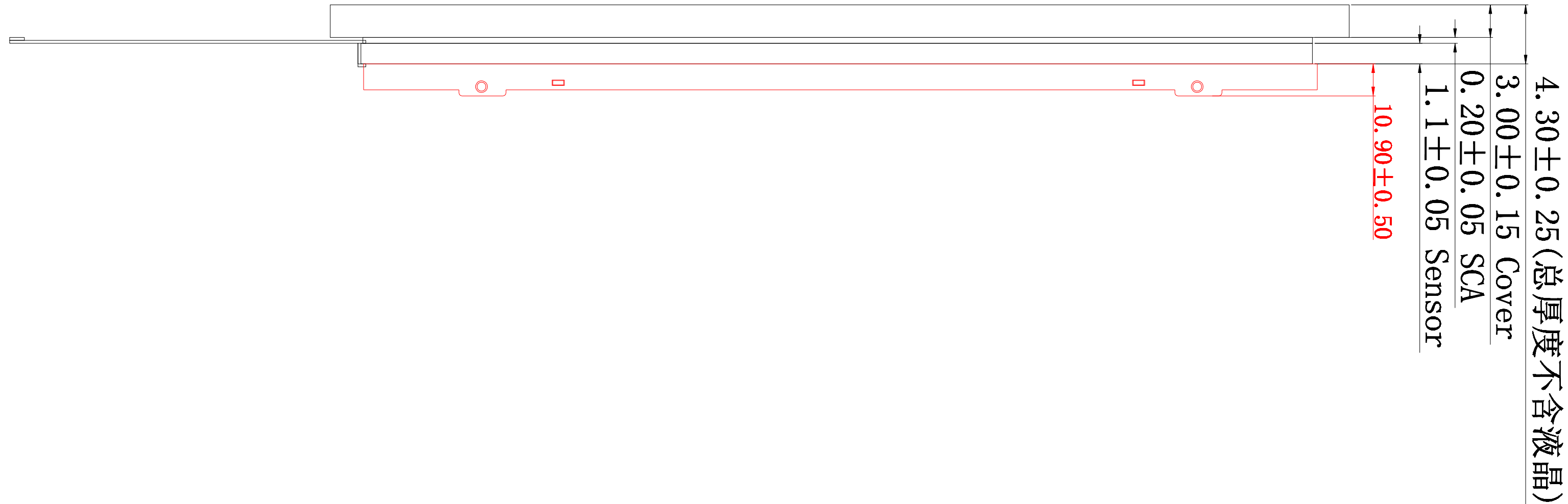
侧视图 横向10:1
