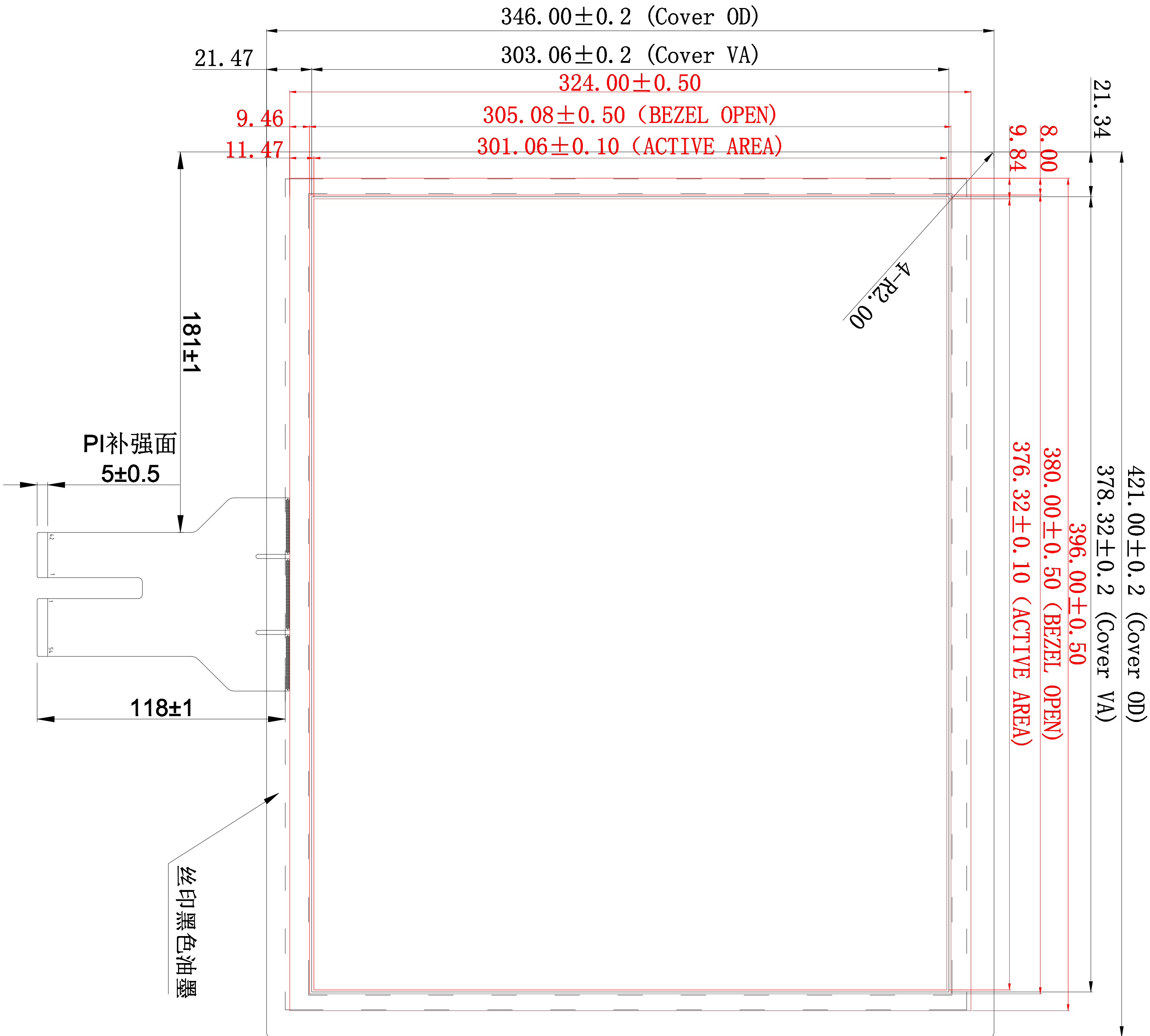
前视图 1:1
