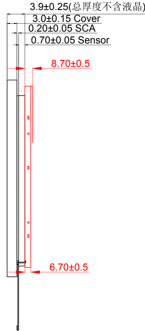
侧视图 横向10:1
