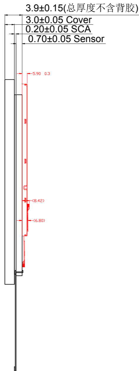
侧视图 横向10:1
