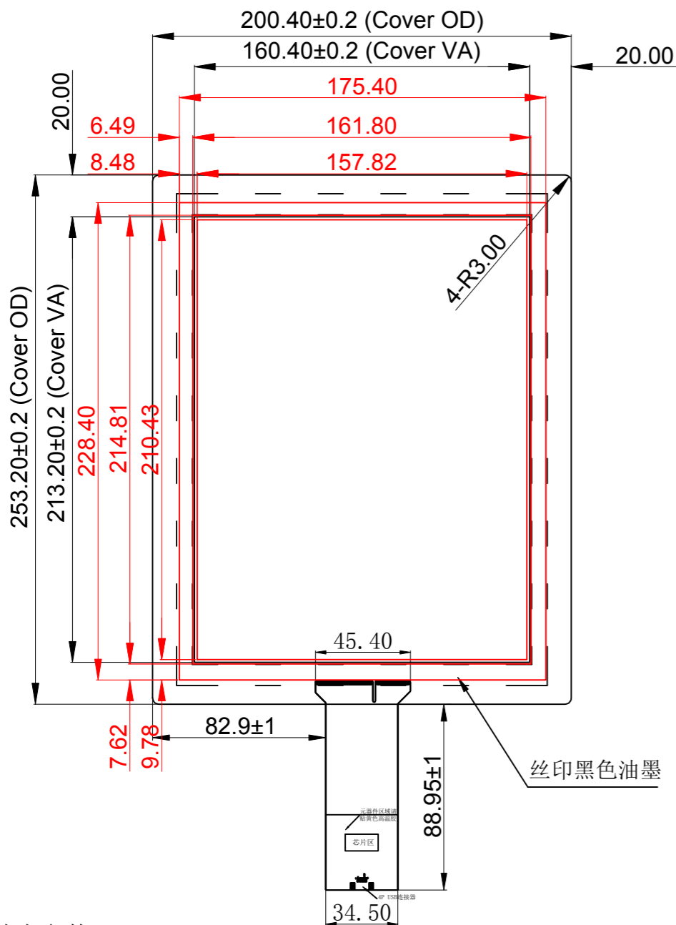
前视图 1:1
